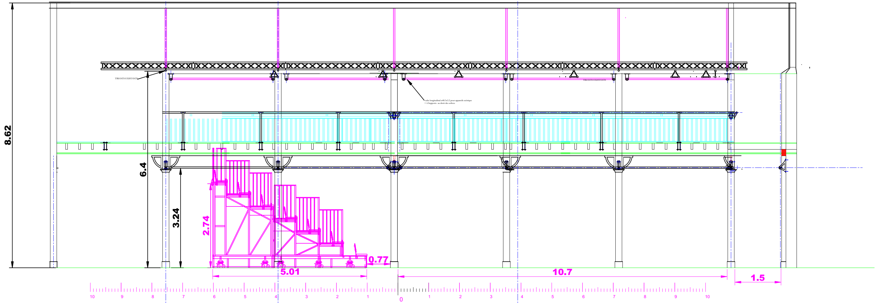
LE GYMNASSE CDCN PLAN DE COUPE LONGITUDINALE
