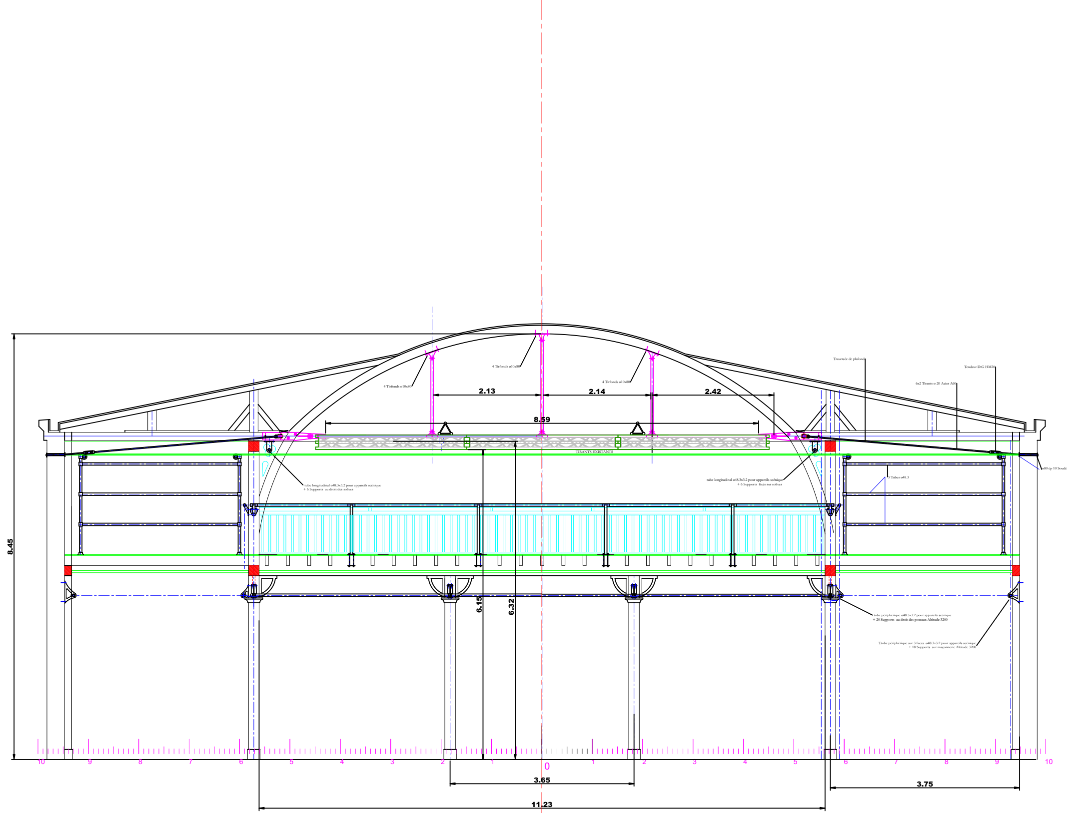
LE GYMNASSE CDCN COUPE TRANSVERSALE
