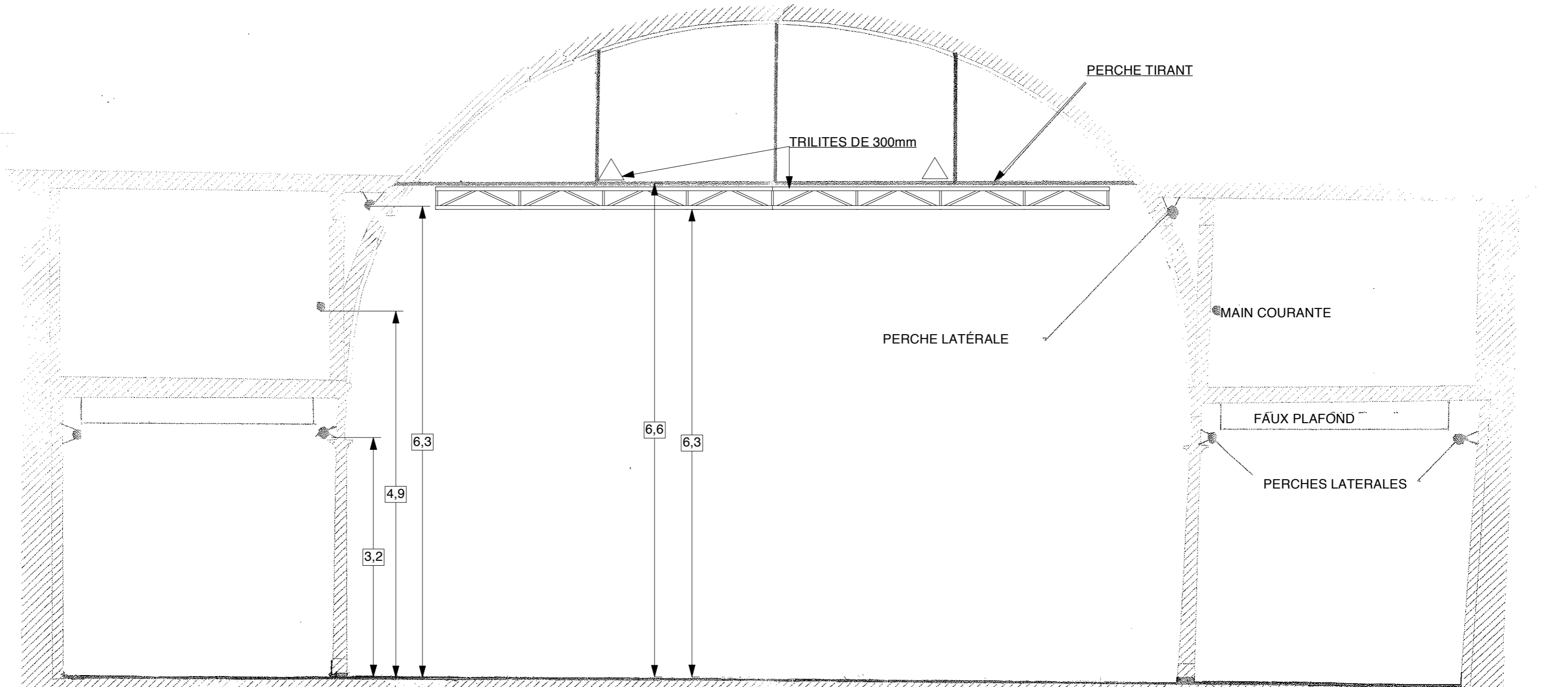
LE GYMNASE- ROUBAIX COUPE LATÉRALE- 1/50e A3
